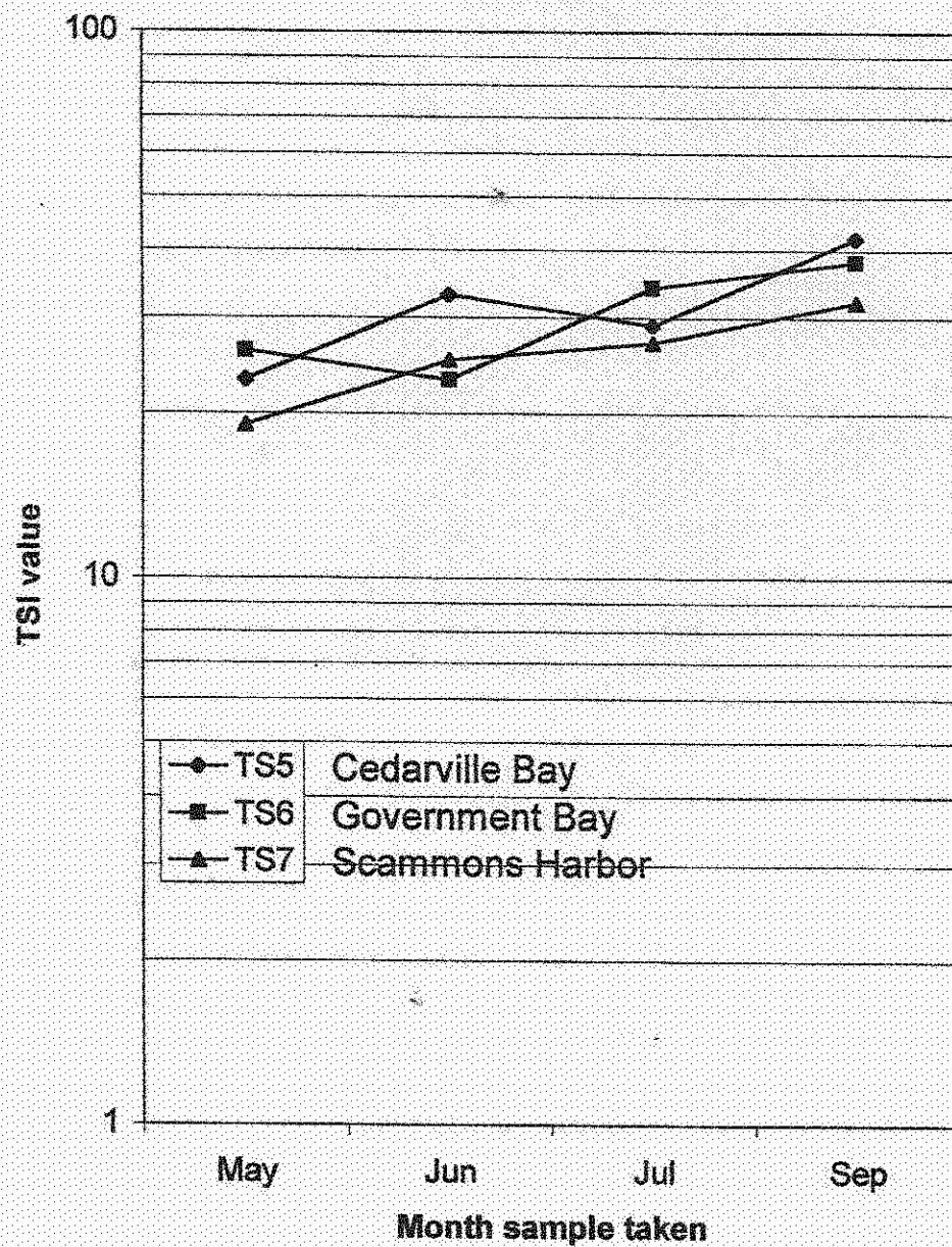
Fig. 5. Chlorophyll TSI values for Les Cheneaux sites TS5, TS6 & TS7, 2001.
